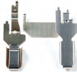
3980524D02 Contacto de batería (-/+) SP50
